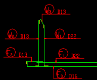
主鉄筋組立図
